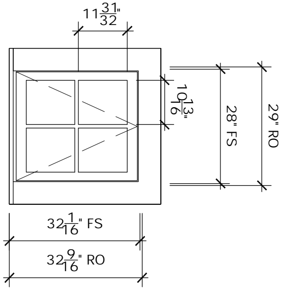
A QTY 3 MAWN 2832 ROTO SCALE: 1/2" = 1'-0" 6-9/16" JAMBS
